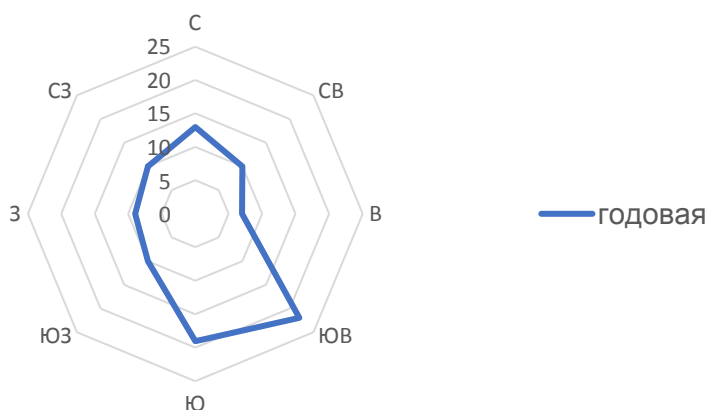
Рисунок 1 - Годовая роза ветров по метеостанции Серноводск
