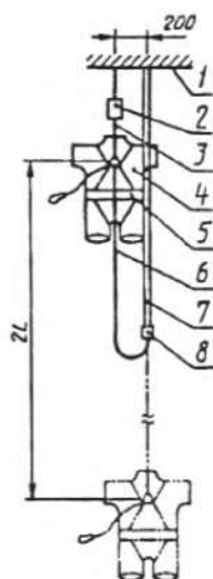
1 – жесткая опора; 2 – сбрасыватель; 3 – соединительное устройство; 4 – манекен; 5 – ляпочный пояс; 6 – строп; 7 – штанга; 8 – серьга штанги;
